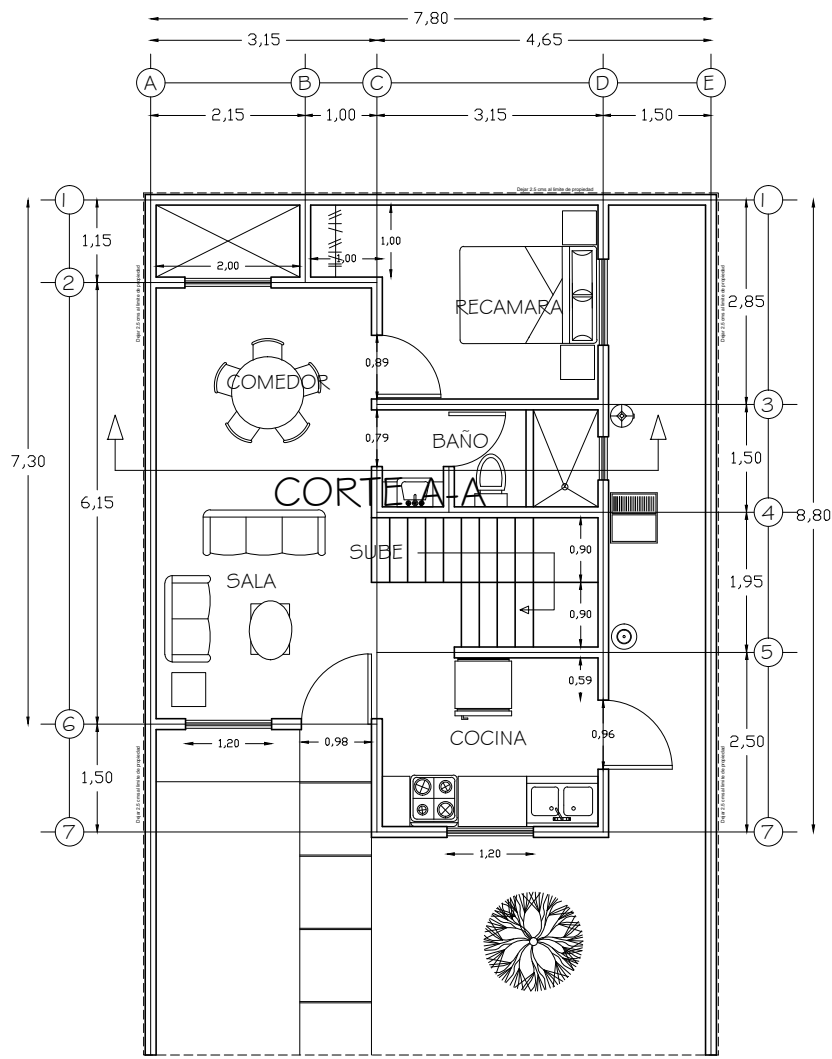
PLANTA BAJA
