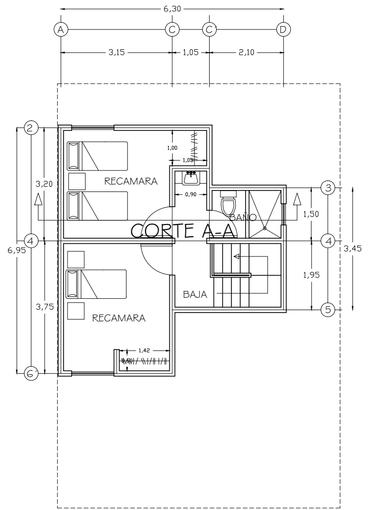
PLANTA ALTA
