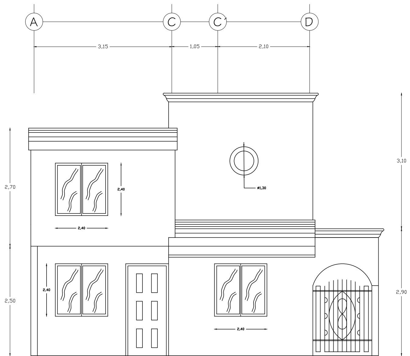
FACHADA
