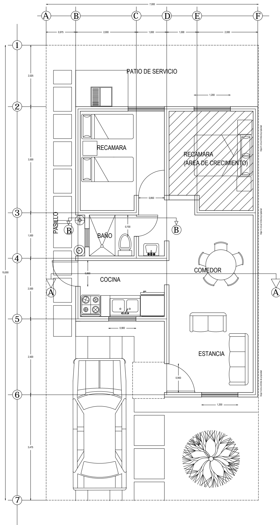
PLANTA ARQUITECTONICA
